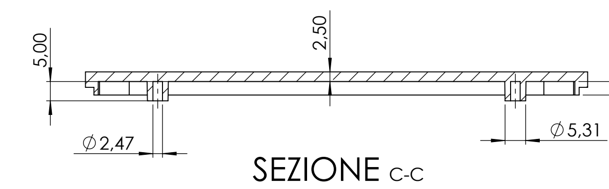
SEZIONE C-C
