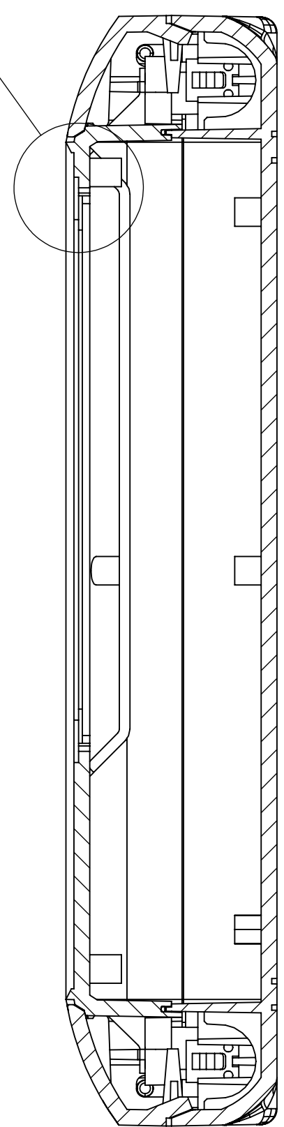
SEZIONE A-A
