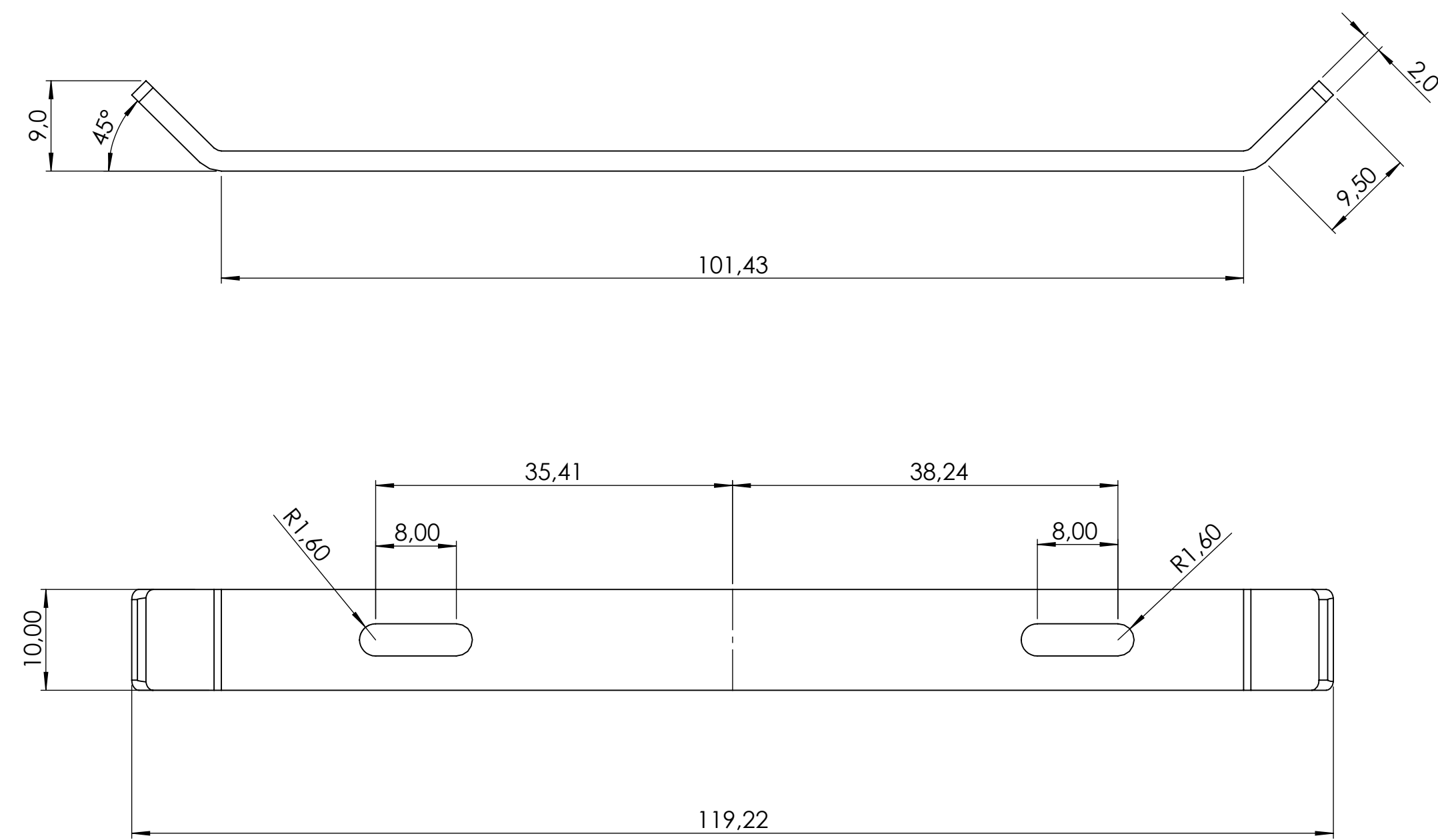
PARTICOLARE SCALA 2:1
