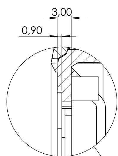
DETTAGLIO B
