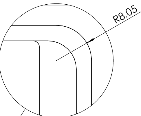
DETTAGLIO C
